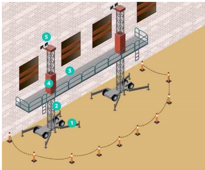
Figur 1 - Arbejdspladsformens primære dele: 1. Bundramme med støtteben 2. Mast 3. Arbejdsstandplads 4. Masteinddækning 5. Forankring af mast
