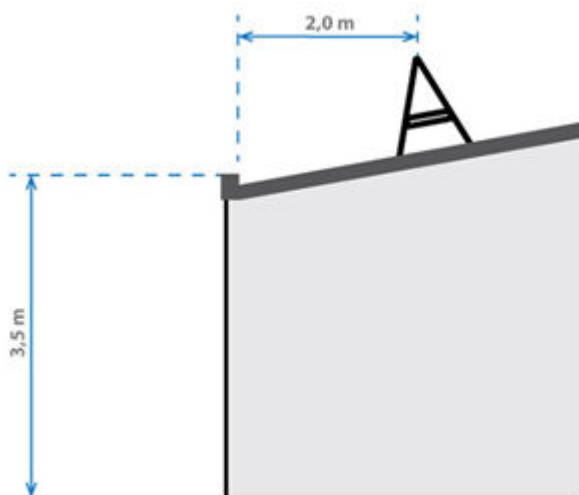
Figur 1.5.3 – Tydelig og holdbar markering placeret to meter fra tagkant.
