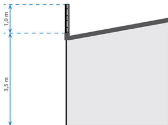
Figur 1.5.1 – Rækværk/skærm placeret som sikring på tagkant.
