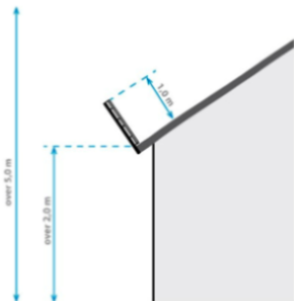
Figur 3.6.1 – Klasse C-skærme placeret som sikring på tagfod og på tagflade. Der kan bruges B-skærme i stedet, hvis den lodrette afstand reduceres til 2 meter.
