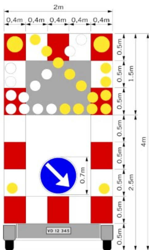
Figur 2. Afspærringsvogn med færdselstavle samt gule blinksignaler, der kan vise blinkende lyspil orienteret mod højre eller mod venstre.
